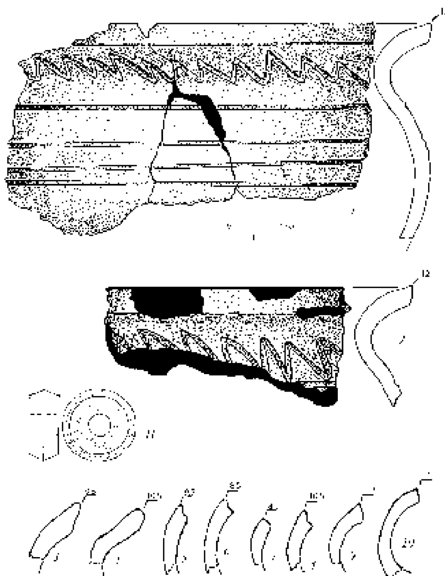
Рис. 4. Великий Дивлин II, «Гора Дивлинська»:
