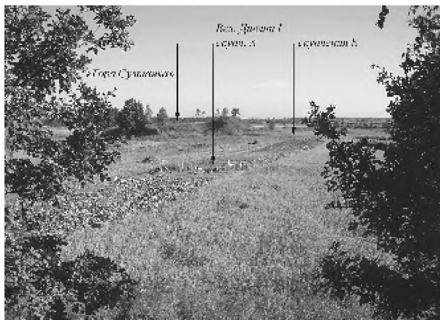
Рис. 2. Загальний вид на комплекс пам'яток з півдня
