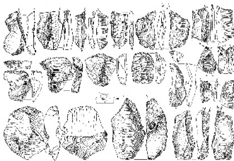
Рис. 3. Великий Дивлин I, скупчення А. Знаряддя праці з кременю
