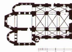
Петропавлівська церква: план і західний фасада (1840-і роки).
